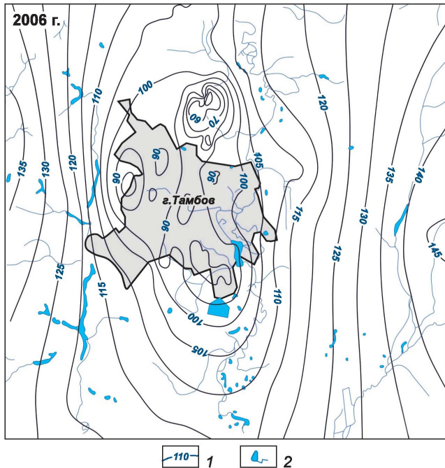
Рис. 1.20. Схема распространения депрессионной воронки в верхнефаменском водоносном горизонте (Филиал ФГУП "Геоцентр-Москва" ТЦ ГМСН и ВО "Тамбовгеомониторинг")
