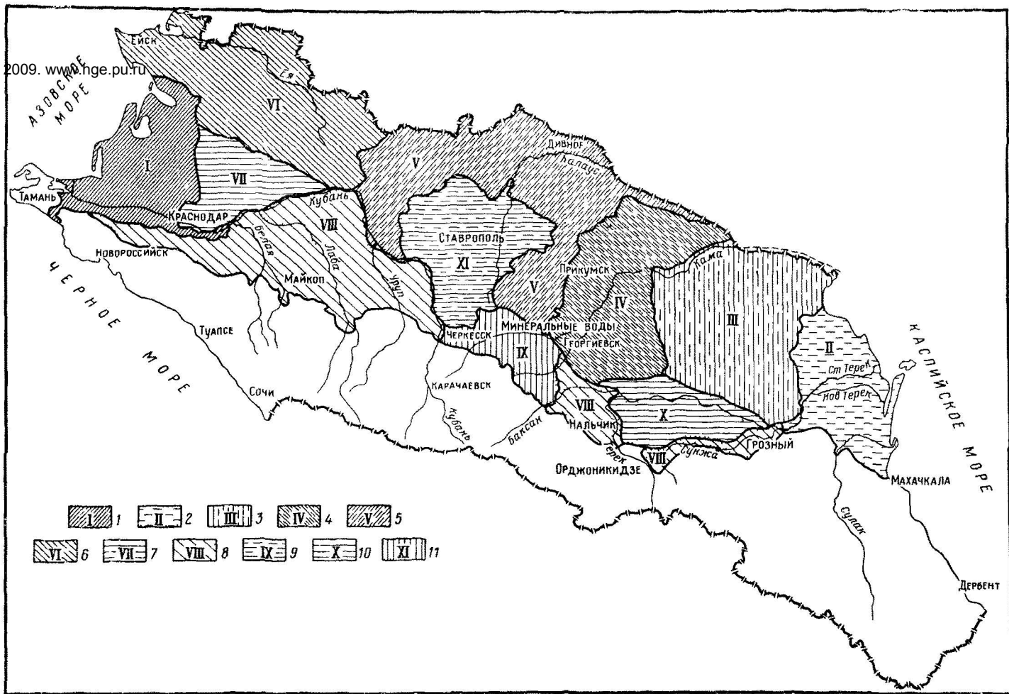
Рис. 39 Схематическая карта гидрогеологического районирования Северного Кавказа (Составил В. С. Щепкин)
