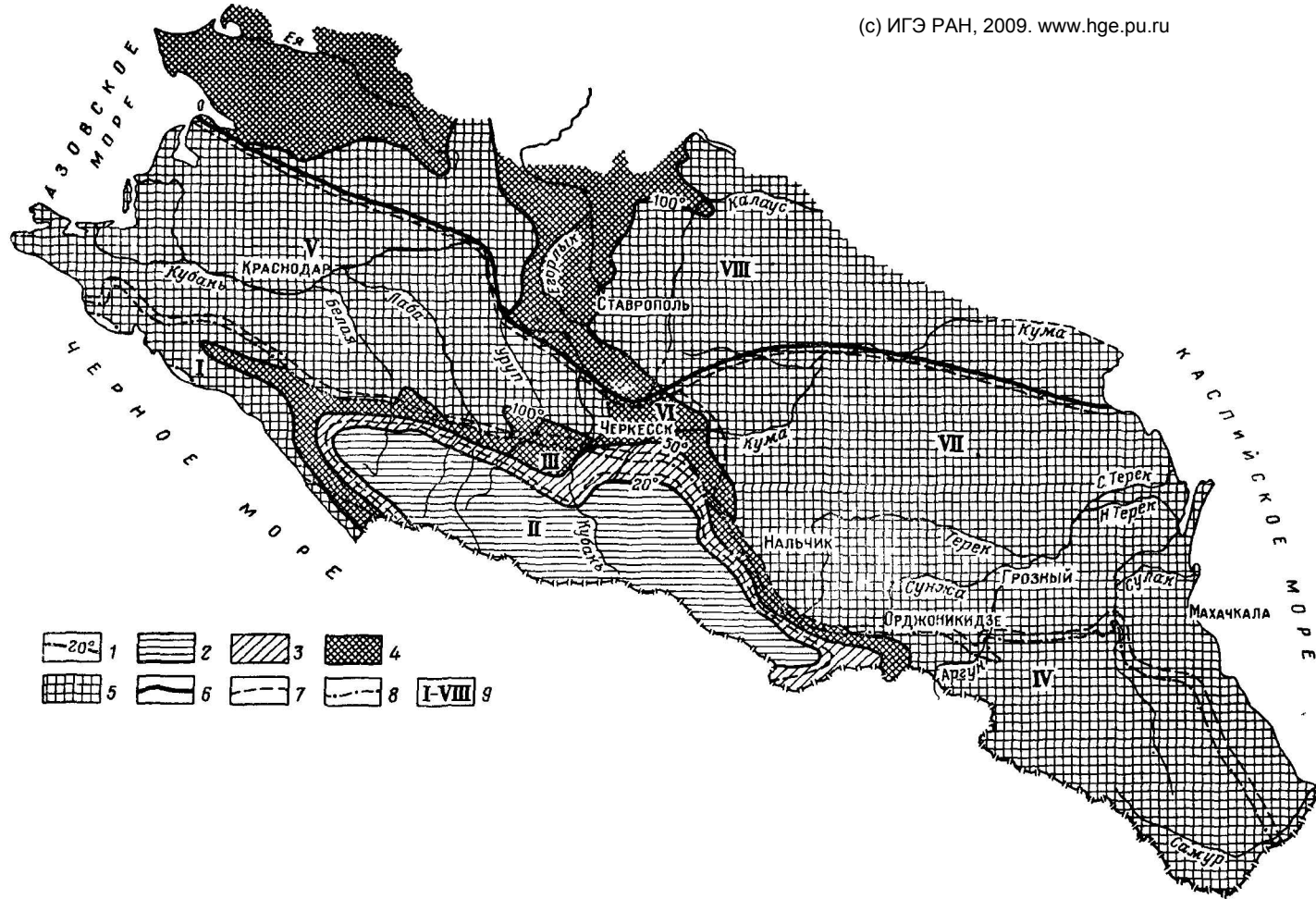
Рис. 30. Схема районирования термальных вод Северного Кавказа (Составил А. И Хребтов)
