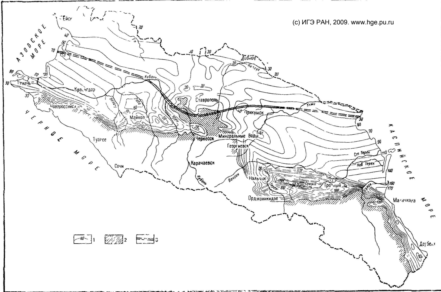
Рис 28 Схемы геонизо терм по поверхности майкопских отложений Северного Кавказа (Составили А И Хребтов, В. С Котов, С. А. Джемалова, Р А Левкович) 1 — геонизотермы в абсолютных отметках, м, 2 — выходы на поверхность майкопских отложений 3 — северная граница районов устойчиво самоизливающихся подземными водами
