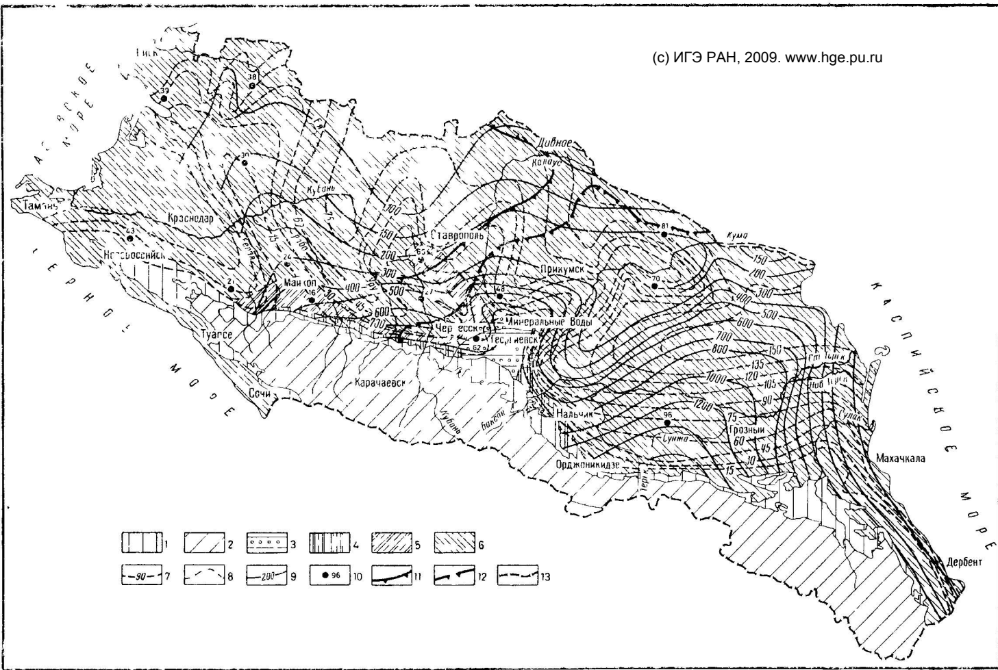
Рис. 22. Схематическая карта пьезозон и химического состава вод отложений нижнего мела (Составили Г. М. Сухарев, Ю. К. Тарануха, Н. С. Погорельский)
