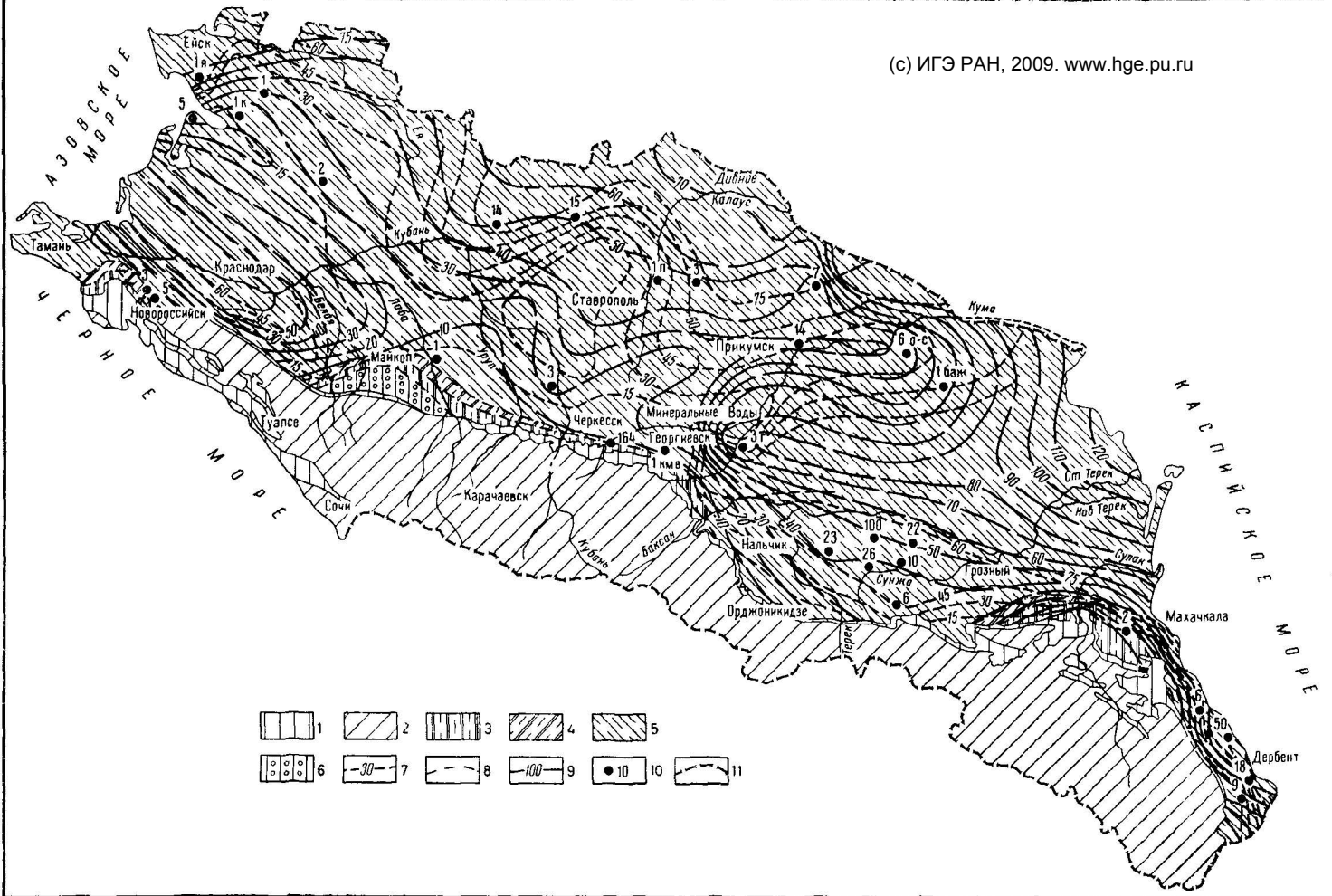
Рис. 21 Схематическая карта пьезоизогипс и химического состава вод в отложениях верхнего мела (Составили Г. М. Сухарев, Ю. К. Тарануха, Н. С. Погорельский)
