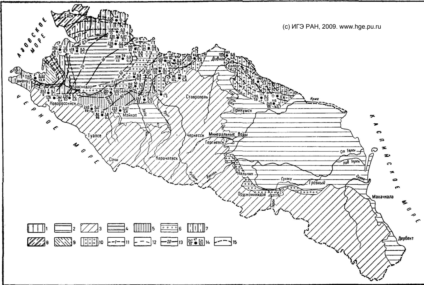
Рис. 12. Схематическая карта пьезоизогипс и химического состава вод отложений понта (Составил Н. С. Погорельский)
