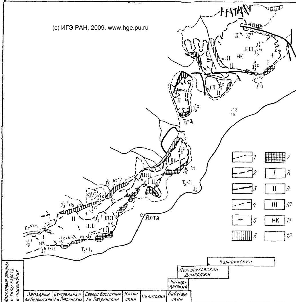
Рис 6 Схематическая карта карстовых районов Горного Крыма Составил Б Н Иванов
