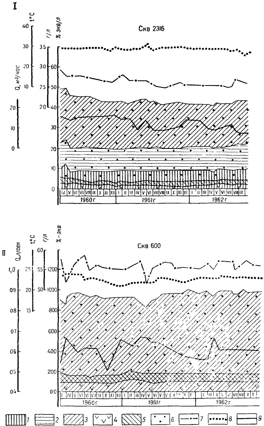
Рис. 82. Графики режимных гидрогеологических наблюдений I — по скв 2316, II — по скв 600, 1—6 содержание компонентов (1 — гидрокарбонатов, 2 — сульфатов, 3 — хлоридов, 4 — кальция, 5 — магния, 6 — натрия), 7 — минерализация, г/л, 8 — температура воды, °С, 9 — дебит, л/сек
