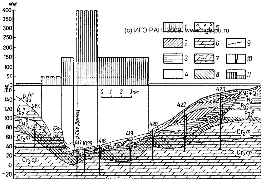
Рис. 78. Схема питания подземных вод мергельно-мелового водоносного горизонта (Ольховский участок долины р. Сев. Донца).
