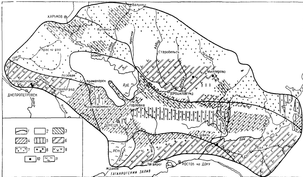
Рис 76 Схематическая карта химического состава и минерализации подземных вод на территории Донбасса на глубине 300 м (Составил Ю Г Головченко)
