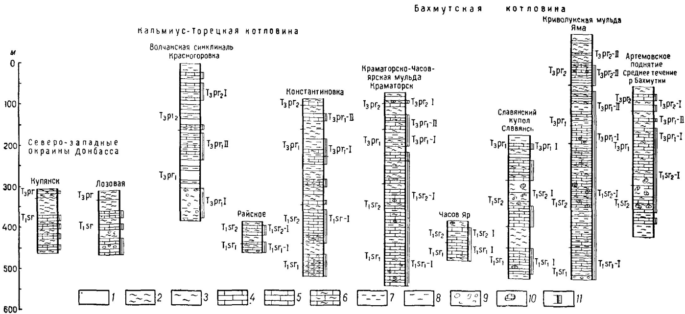
Рис. 38. Сопоставление водоносных горизонтов триасовых отложений
