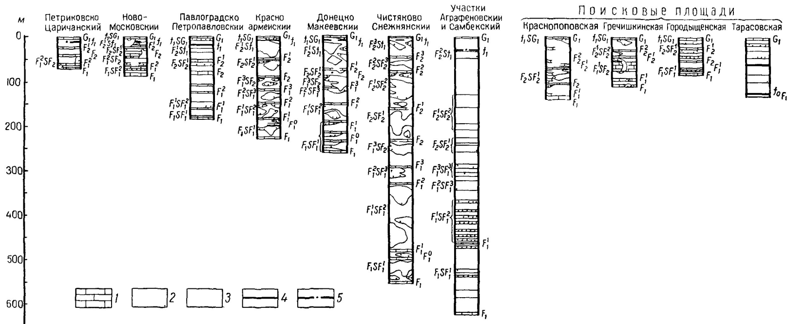
Рис 20 Сопоставление водоносных горизонтов свиты C_2^1
