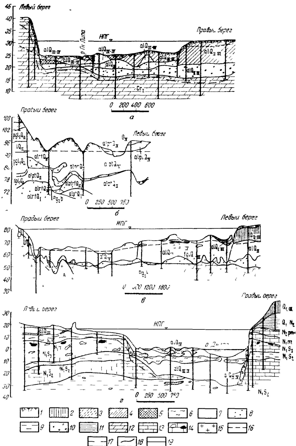
Рис 92 Геолого-литологические профили по створам плотин
