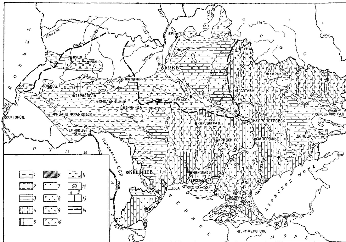
Рис. 85. Карта мощностей и состава лёссовых пород УССР. Составил В. Ф. Краев
