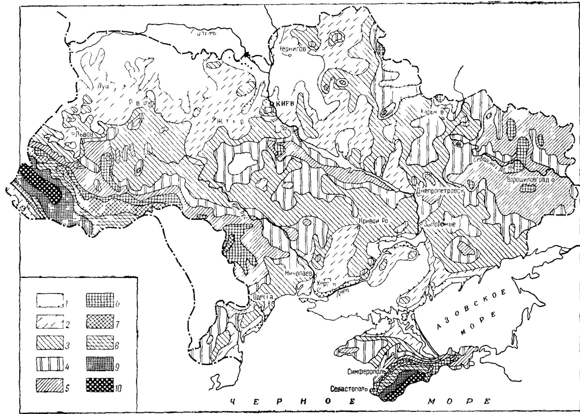
Рис 73. Карта глубин расчленения поверхности Составил В М Чернин
