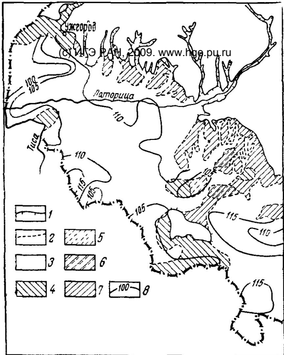
Рис. 54. Схематическая карта распространения и глубин залегания водоносного горизонта в аллювиальных отложениях Чоп-Мукачевского артезианского бассейна
