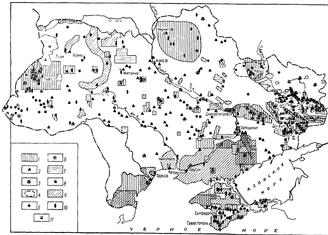
Рис. 1. Карта гидрогеологической изученности территории Украинской ССР (составила Т. Д. Найденова)
