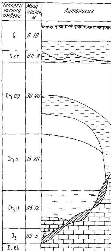
Рис 98 Стратиграфическая колонка района Липецких железорудных месторождений По Г Я Борисенкову и В П. Орешкину
