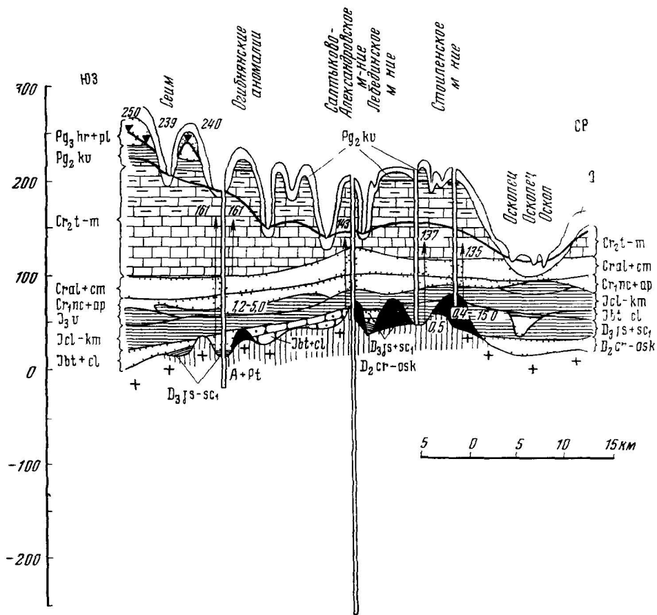
Рис 80 Гидрогеологический разрез вкостр простираения рудных залежей железо рудных месторождений КМА старооскольского типа Составил Б Н Смирнов Условные обозначения см на рис 74
