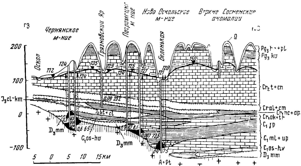
Рис 78 Гидрогеологический разрез по простиранию рудных залежей железорудных месторождений КМА новооскольского типа Составил Б Н Смирнов Условные обозначения см на рис 74
