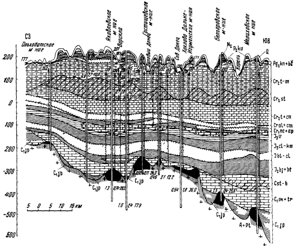
Рис 75 Гидрогеологический разрез по простиранию рудных залежей железорудных месторождений КМА белгородского типа Составил Б Н Смирнов Условные обозначения см на рис 74
