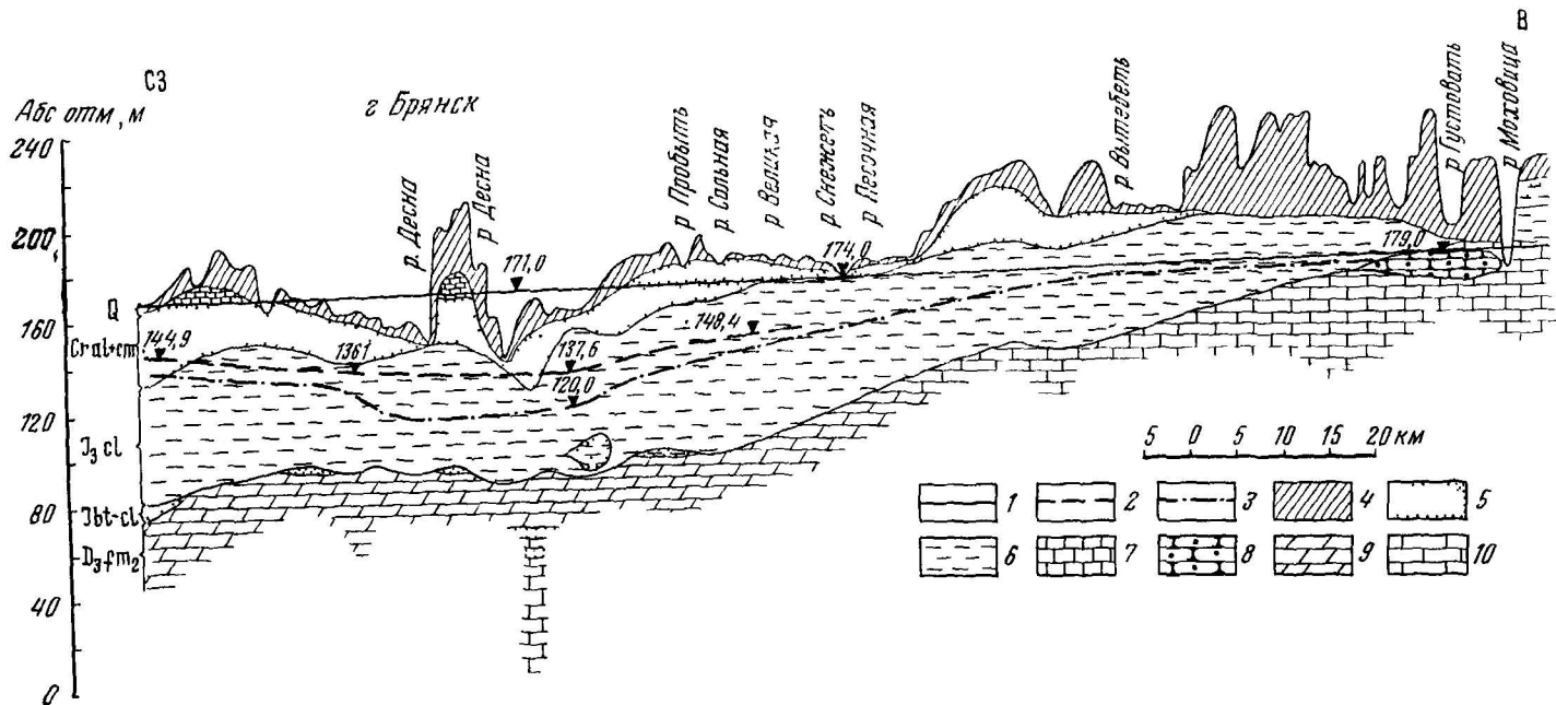
Рис 64 Гидрогеологический разрез через район Брянского водозабора Составил В. С. Плотников и др. Уровни воды верхнедевонского водоносного комплекса (в абсолютных отметках) 1 — статический (1928 г.) 2 — динамический (в 1964 г.), 3 — прогнозный (на 1980 г.) 4 — суглинки, 5 — пески 6 — глины 7 — мел 8 — песчаники 9 — доломиты 10 — известняки
