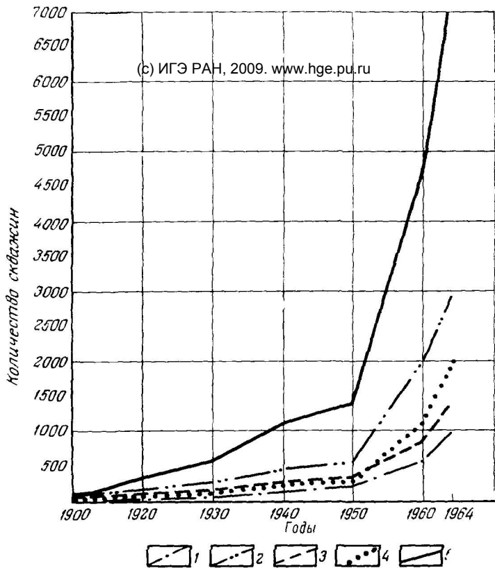
Рис 54 Рост количества действующих водозаборных скважин. Составил В. С. Плотников
