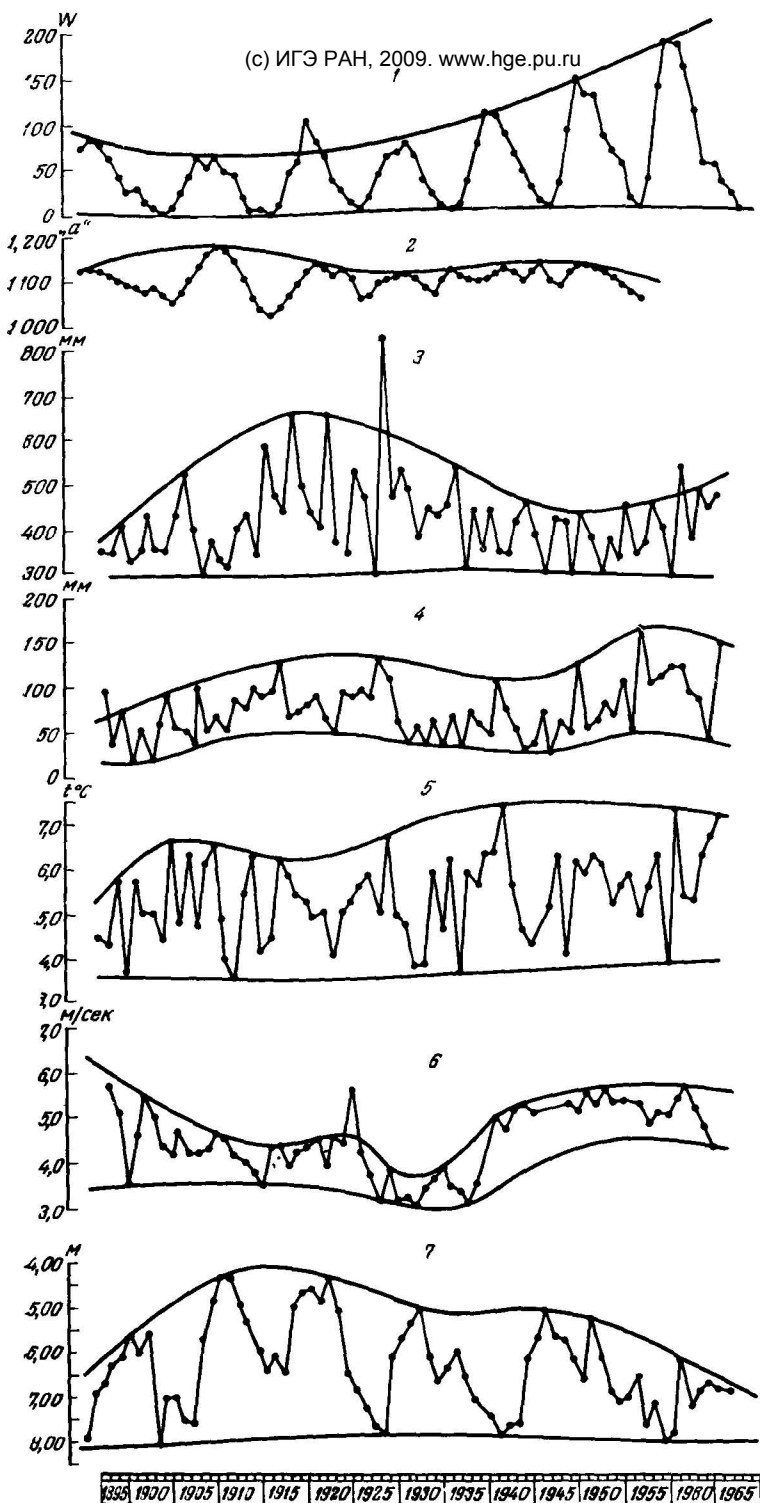
Рис 46 Хронологические графики изменений природных процессов, влияющих на уровень грунтовых вод. Составил В. А. Коробейников
