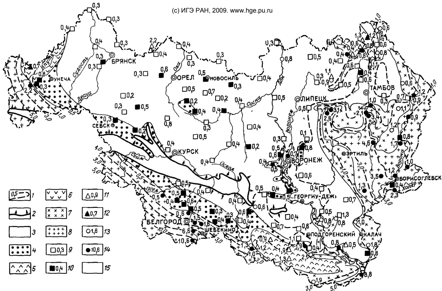
Рис. 34. Гидрохимическая карта первых от поверхности водоносных горизонтов палеозоя. Составил Б. Н. Смирнов
