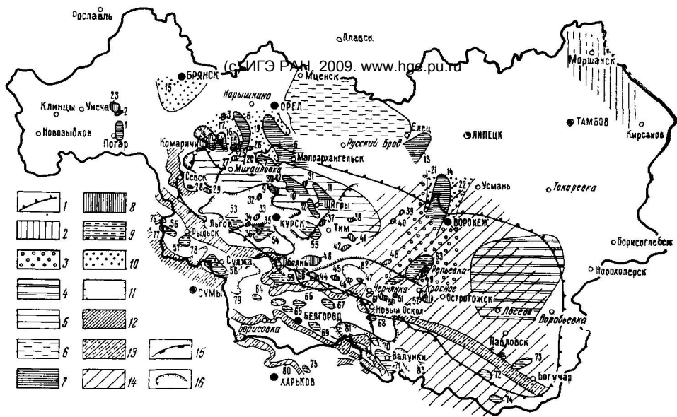
Рис. 12. Схема тектоники осадочной толщи Воронежской антеклизы. Составил Д. Н. Утехин
