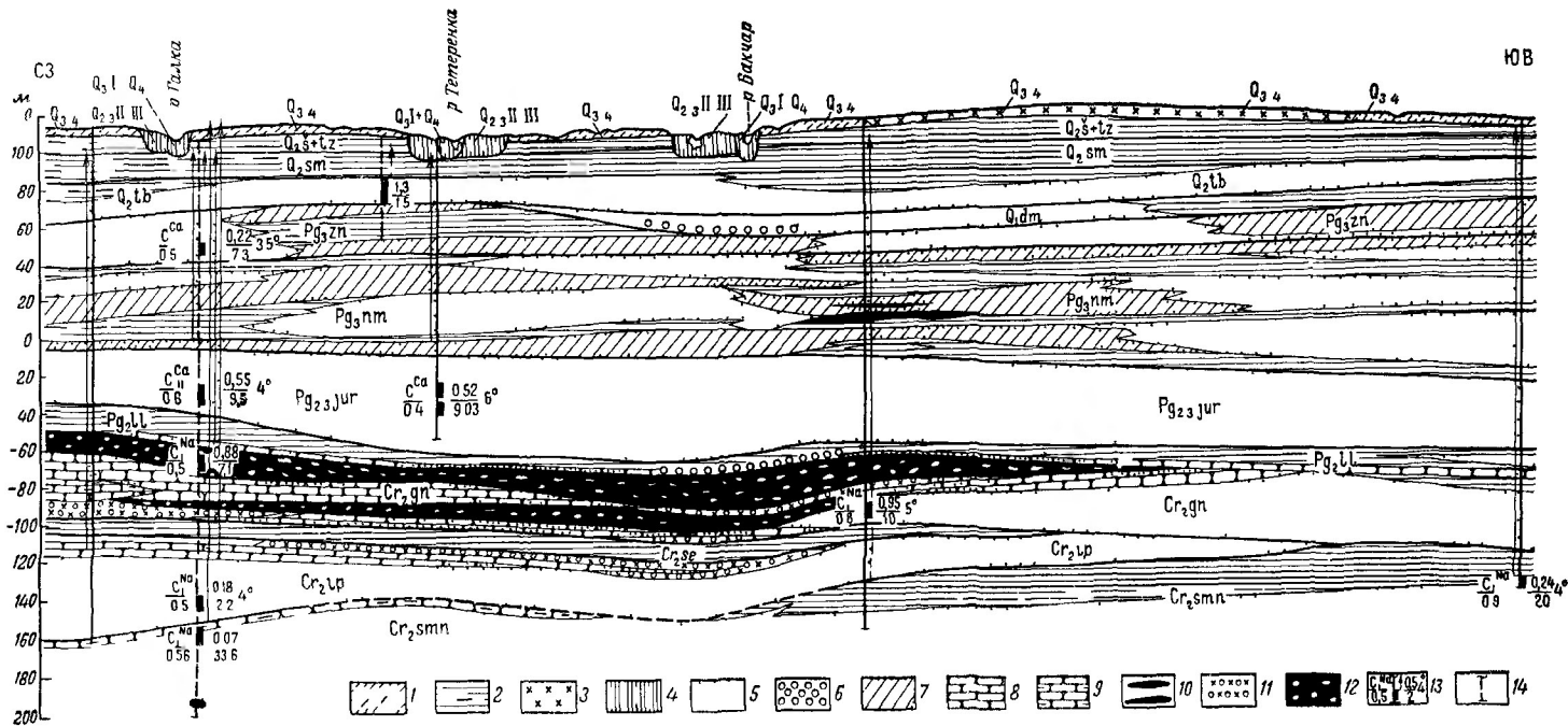
Рис 63 Схематический гидрогеологический разрез Бакcharsкого железорудного месторождения (составили А А Бабин и О А Гусельникова) 1 — суглинки 2 — глины 3 — торф 4 — переслаивание глин суглинков песков супесей 5 — пески 6 — галечники 7 — алевроиты 8 — песчаники 9 — алевролиты 10 — бурые или лигниты 11 — песчаники железистые оолитовые оруденелые 12 — оолитовые железные руды 13 — скважина или тервал опробования (стрелка — напор подземных вод слева в числителе — тип воды по О А Алексиу в знаменателе — минерализация воды г/л (справа в числителе — удельный дебит л/сек м в знаменателе — понижение м сбоку — температура воды °С 14 — скважина, спроектированная на линию разреза
