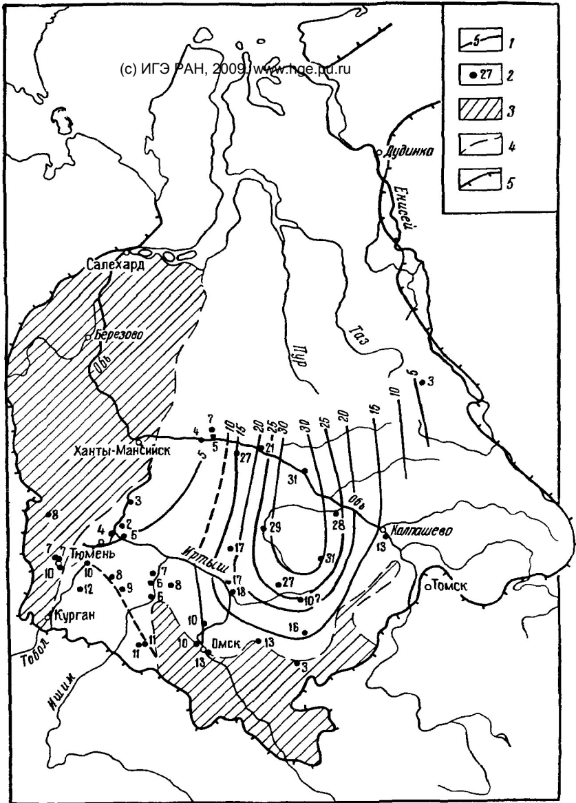
Рис. 31. Изменение содержания иона-кальция в водах нижней части гостерив-барремских отложений, экв. % (составили Б. П. Ставицкий, А. А. Розин)
