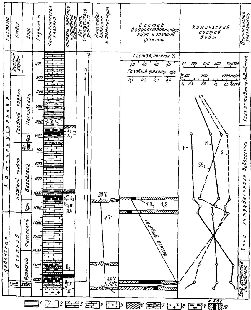
Рис. 85. Сводный гидрогеологический разрез Зольиенского месторождения 1 — аргиллиты; 2 — пески; 3 — мергели; 4 — известняки; 5 — доломиты; 6 — алевролиты; 7 — глинистость; 8 — кристаллический фундамент; 9 — нефтеносные породы; 10 — состав водорастворенного газа в объем %: а — \text{CH}_4 , б — \text{C}_n\text{H}_{2n+2} ; в — кислые газы ( \text{CO}_2 ; \text{H}_2\text{S} ; \text{H}_2 ); г — \text{N}_2 + редкие
