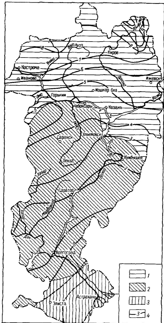
Рис. 66. Карта среднего годового стока рек СССР (Поволжье и Прикамье)
