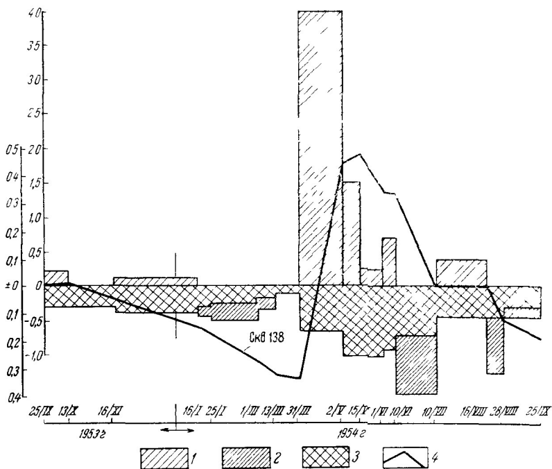
Рис. 52. Динамика элементов баланса грунтовых вод в долине р. Черемшана 1 — инфильтрация атмосферных осадков и вод временного поверхностного стока, 2 — испарение грунтовых вод; 3 — разница между боковым притоком и оттоком грунтовых вод, 4 — колебания уровня грунтовых вод
