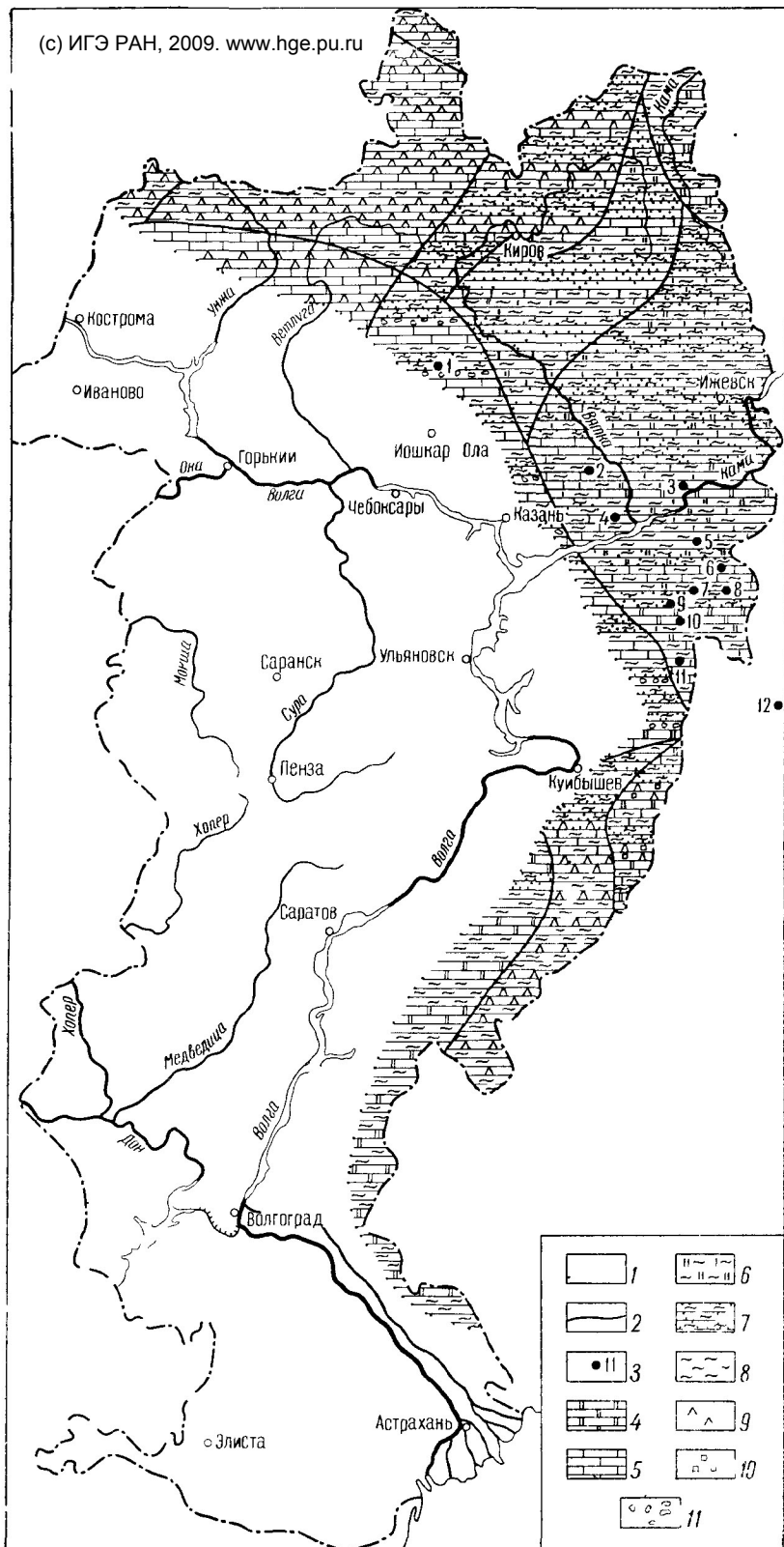
Рис. 41. Схематическая карта распространения подземных вод уфимских отложений 1 — граница распространения уфимских отложений, 2 — литолого-фациальные границы 3 — скважина и ее номер 4 — доломит 5 — известняк 6 — глинистый доломит 7 — глинистый песок песчаник и песчанистая глина 8 — глина 9 — гипс ангидрит 10 — каменная соль 11 — брекчия
