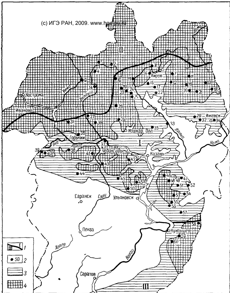
Рис 37 Схема гидрогеологического районирования подземных вод татарских отложений Поволжья и Прикамья 1 — границы гидрогеологических районов (I — центральный II — северный III — южный), 2 — скважина и ее номер, 3 — воды нижнетатарских отложений 4 — воды верхне и ниже татарских отложений
