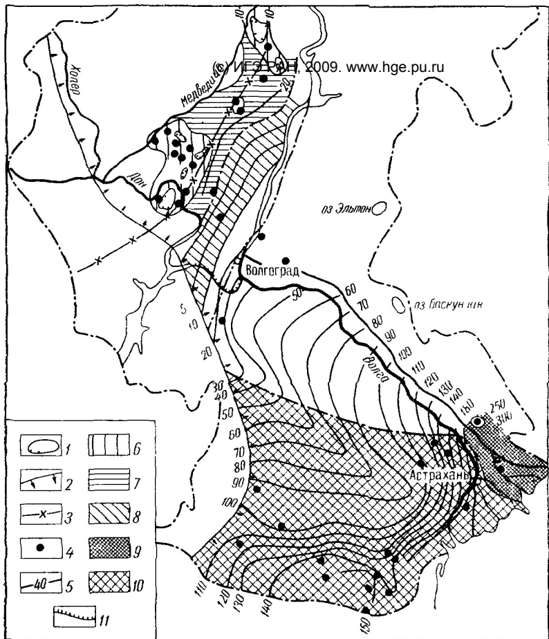
Рис 35. Схематическая гидрохимическая карта байковского водоносного горизонта Волгоградской и Астраханской областей и Калмыцкой АССР. Составила Н. Д. Козлова
