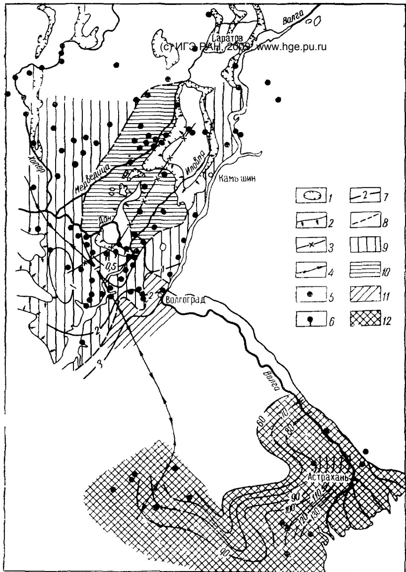
Рис 34 Схематическая гидрохимическая карта альб сеноманского водоносного горизонта Среднего Дона и Нижнего Поволжья Составила Н Д Козлова
