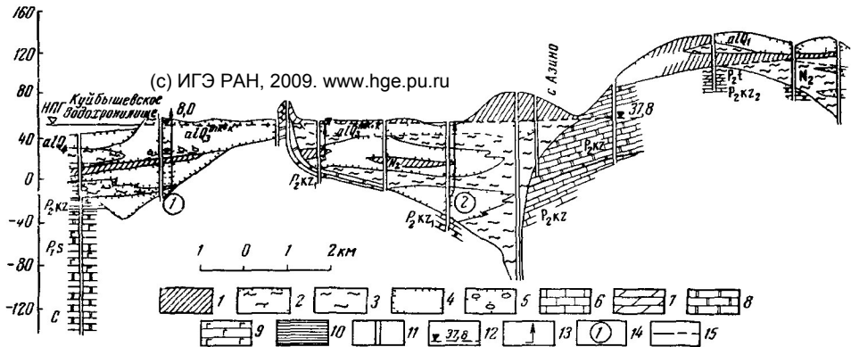
Рис. 28. Гидрогеологический разрез района Казани и сопредельных площадей
