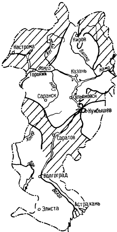
Рис. 10 Распространение додевонских отложений (показано штриховкой)
