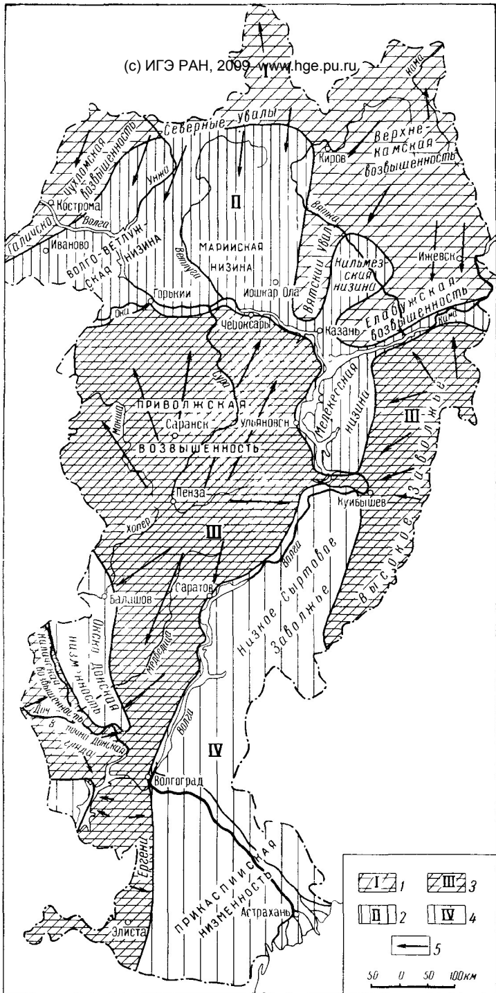
Рис. 3. Орографическая схема
