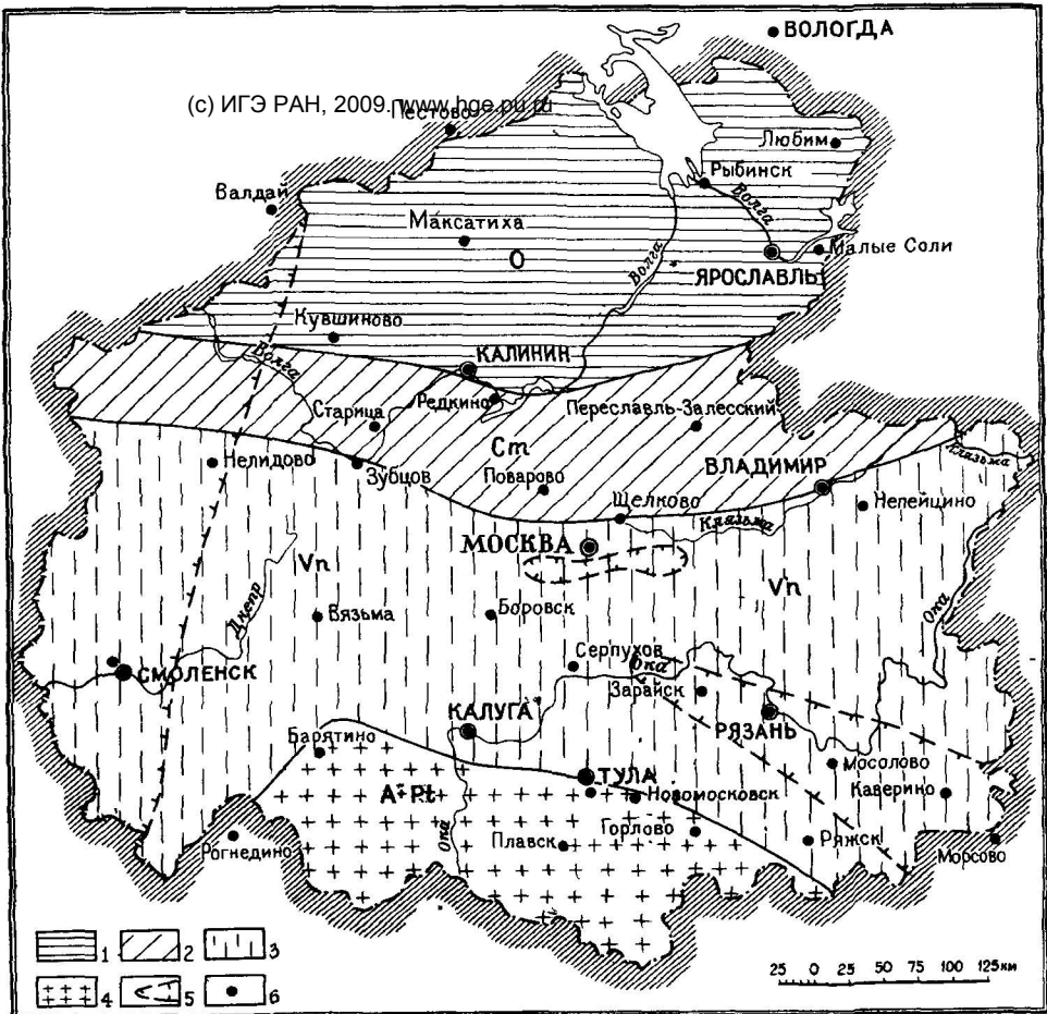
Рис 8 Схематическая геологическая карта додевонских отложений. Составил С. М. Шик
