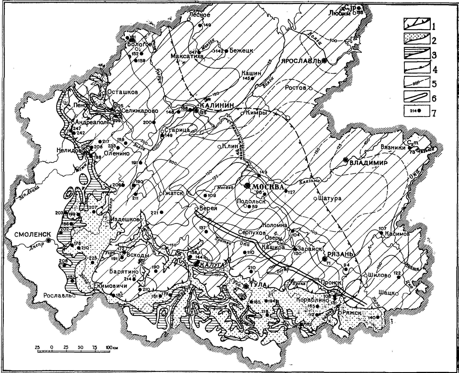
Рис. 28. Карта изопьез первых от поверхности водоносных горизонтов нижнего карбоната. Составили Б. Н. Смирнов и Н. В. Бастракова границы и площади распространения водоносных горизонтов: 1 — серпуховско-окского и протвинского, 2 — яснополянско-го, 3 — упинского (на западе — спорадически распространено в турнейских отложениях), 4 — северо-восточная предполагаемая граница распространения малевских глин, примерно совпадающая с границей упинского водоносного горизонта, 5 — изопьезы протвинского и серпуховско-окского водоносных горизонтов (пунктир — предполагаемые), 6 — доверейская долина, 7 — скважина и абсолютная отметка пьезометрического уровня в ней
