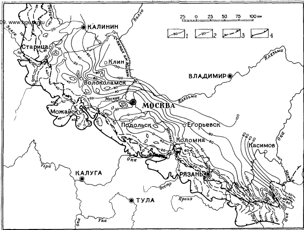
Рис 26 Карта напоров над кровлей среднекаменноугольных водоносных горизонтов (по материалам Подмосковной партии Гидрорежимной экспедиции ВСЕГИНГЕО, 1962 г.)
