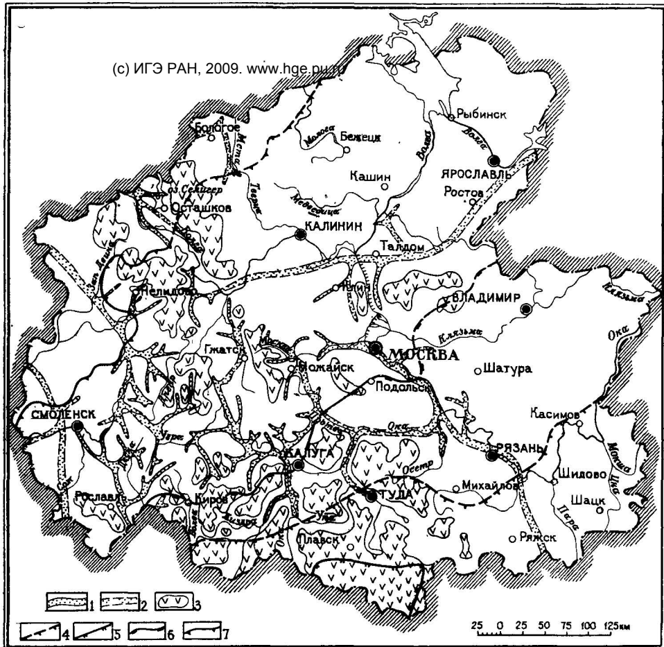
Рис. 11. Схема доледникового рельефа и границ оледенений. Составил С. М. Шик Погребенные доледниковые долины: 1 — прослеженные по данным бурения, 2 — предполагаемые, 3 — водораздельные пространства (с абсолютной высотой кровли дочетвергичных отложений более 200 м). Границы оледенений (сплошные линии — установленные, пунктир — предполагаемые): 4 — окского, 5 — днепровского, 6 — московского, 7 — валдайского
